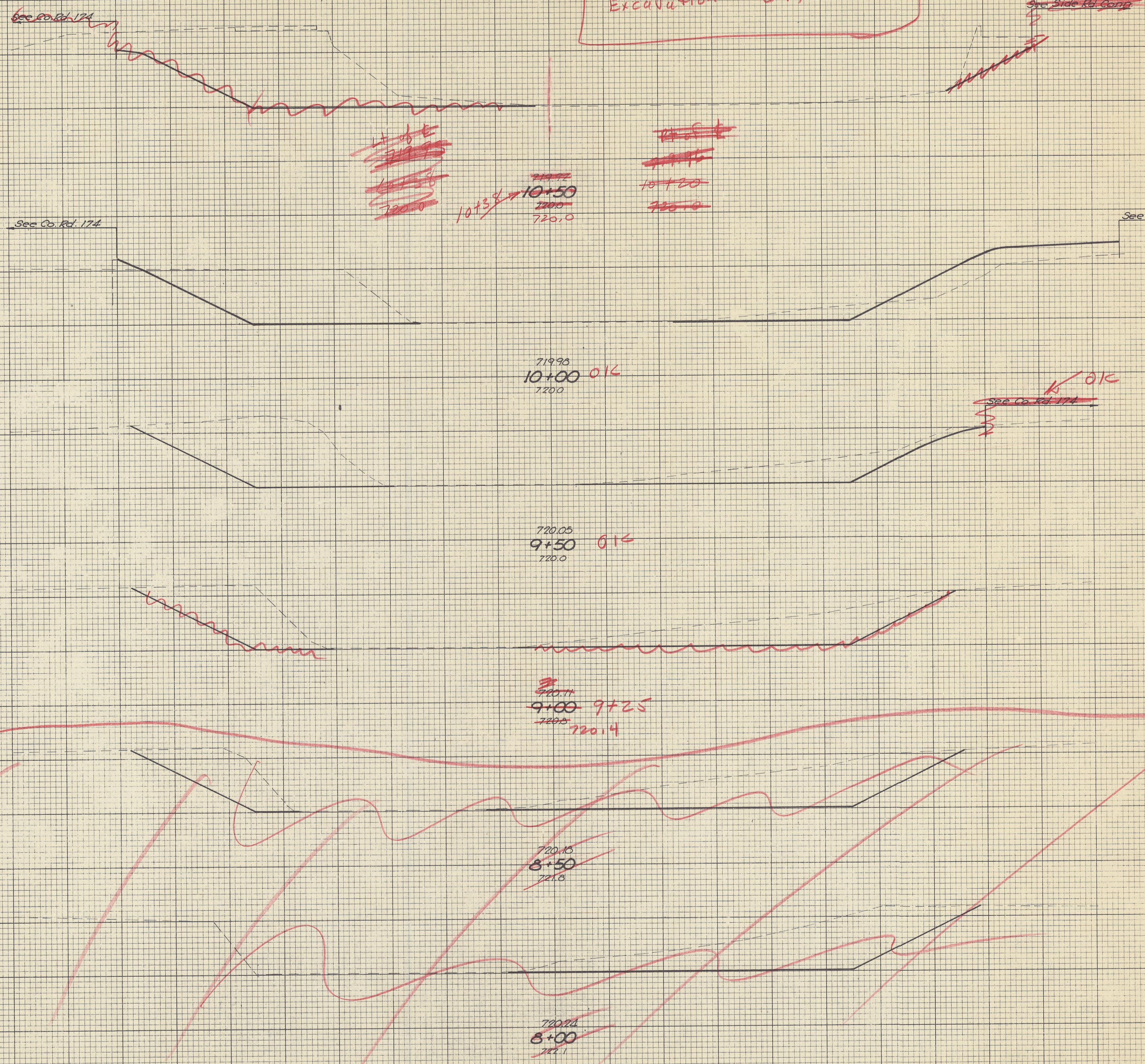
CHANNEL SECTIONS - STA. 8+00 TO STA. 10+50
