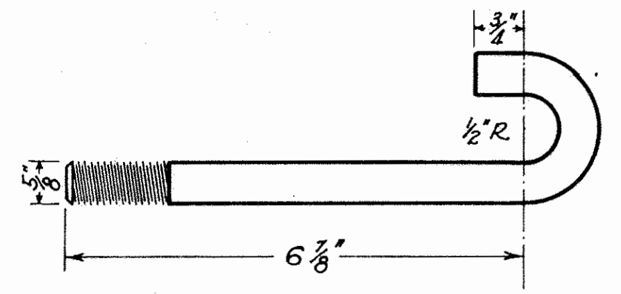
J BOLT
